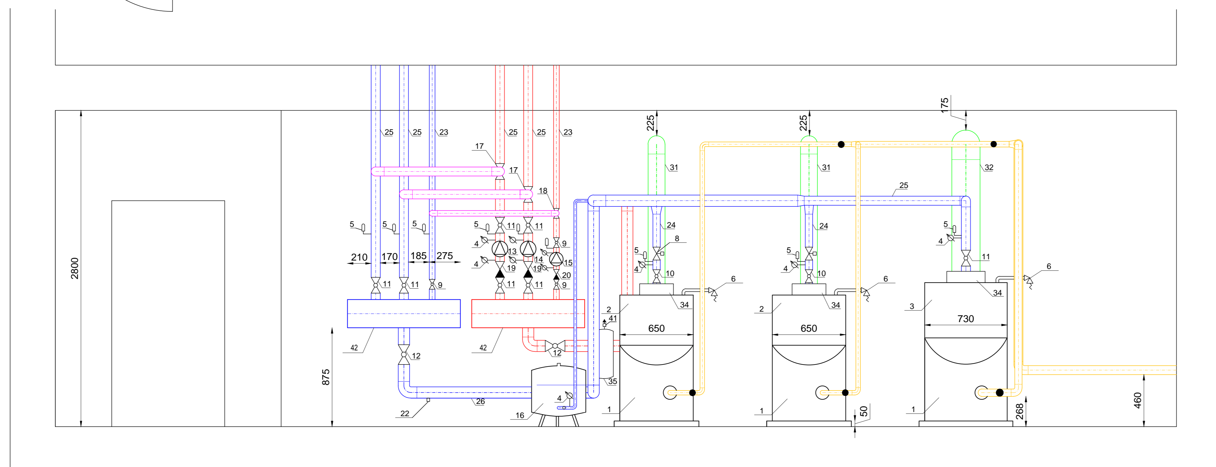
Section A-A
