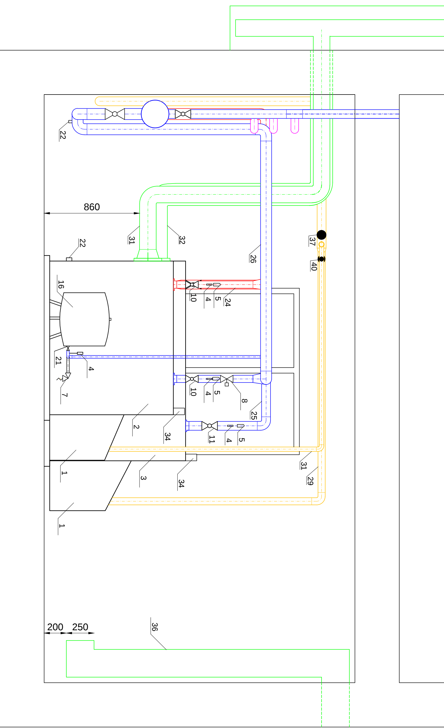
Przekrój B-B
