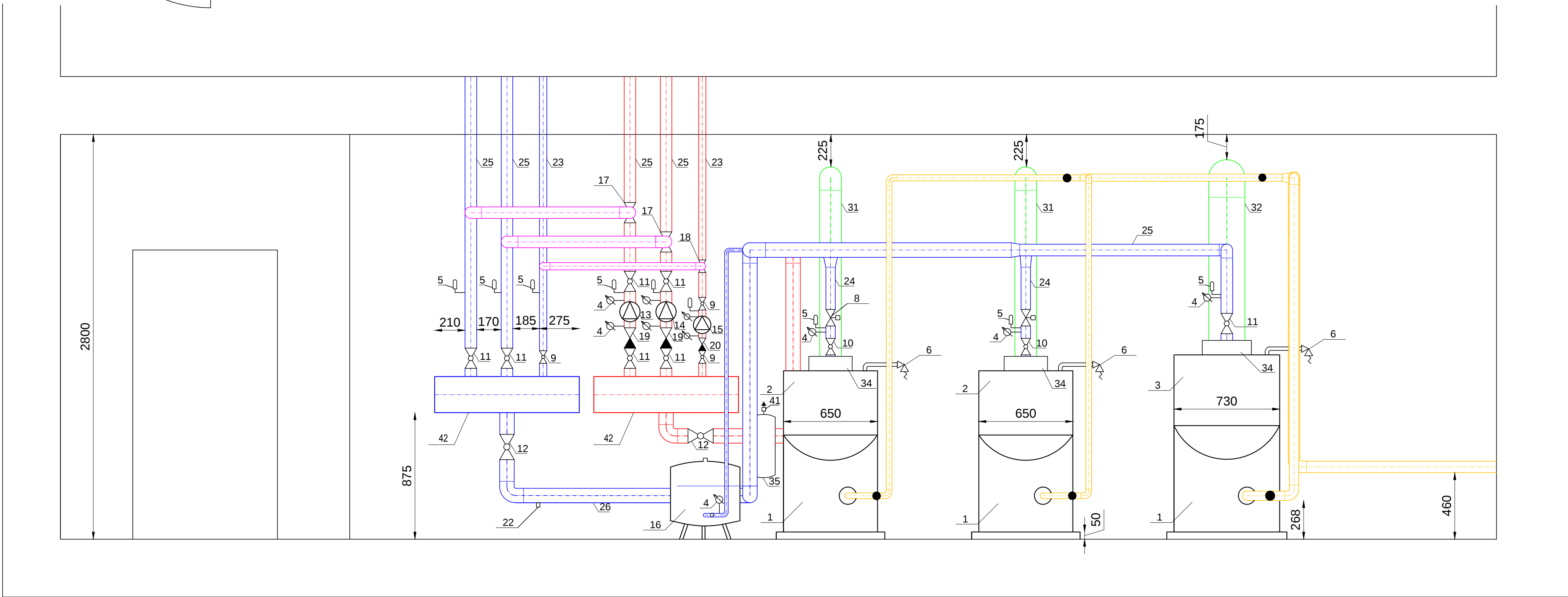
Przekrój A-A
